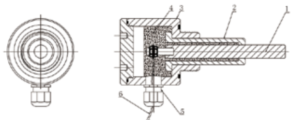
1-高纯锌参比电极；2-PVC护套；3-接合金；4-环氧树脂；5-电缆密封接头；6-电缆
